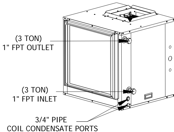
1 TON 2 TON 3 TON HSS® AIR HANDLER PIPING CONNECTIONS
